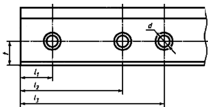
Рисунок 2 - Расположение болтовых отверстий
