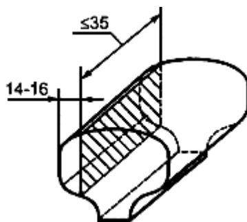
Рисунок 3 - Схема вырезки микрошлифа
