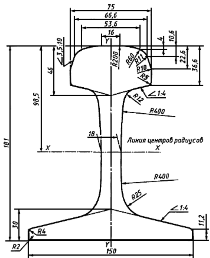
Рисунок А.3 - Рельс типа Р65К
